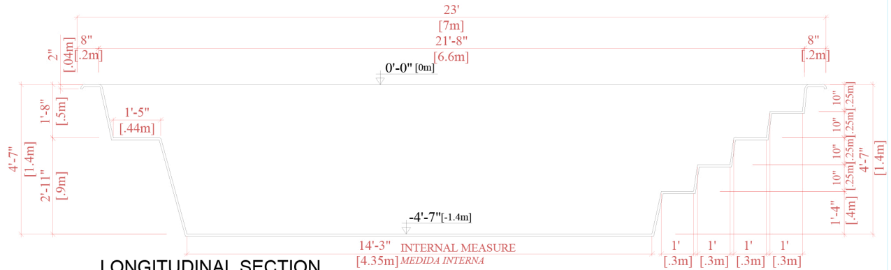
LONGITUDINAL SECTION CORTE LONGITUDINAL
