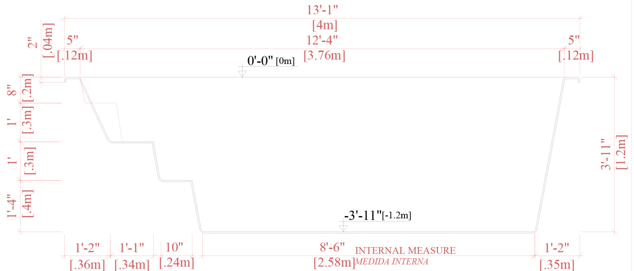
LONGITUDINAL SECTION CORTE LONGITUDINAL
